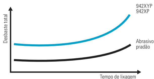
Lixagem de bobines e chapas finas de aço
